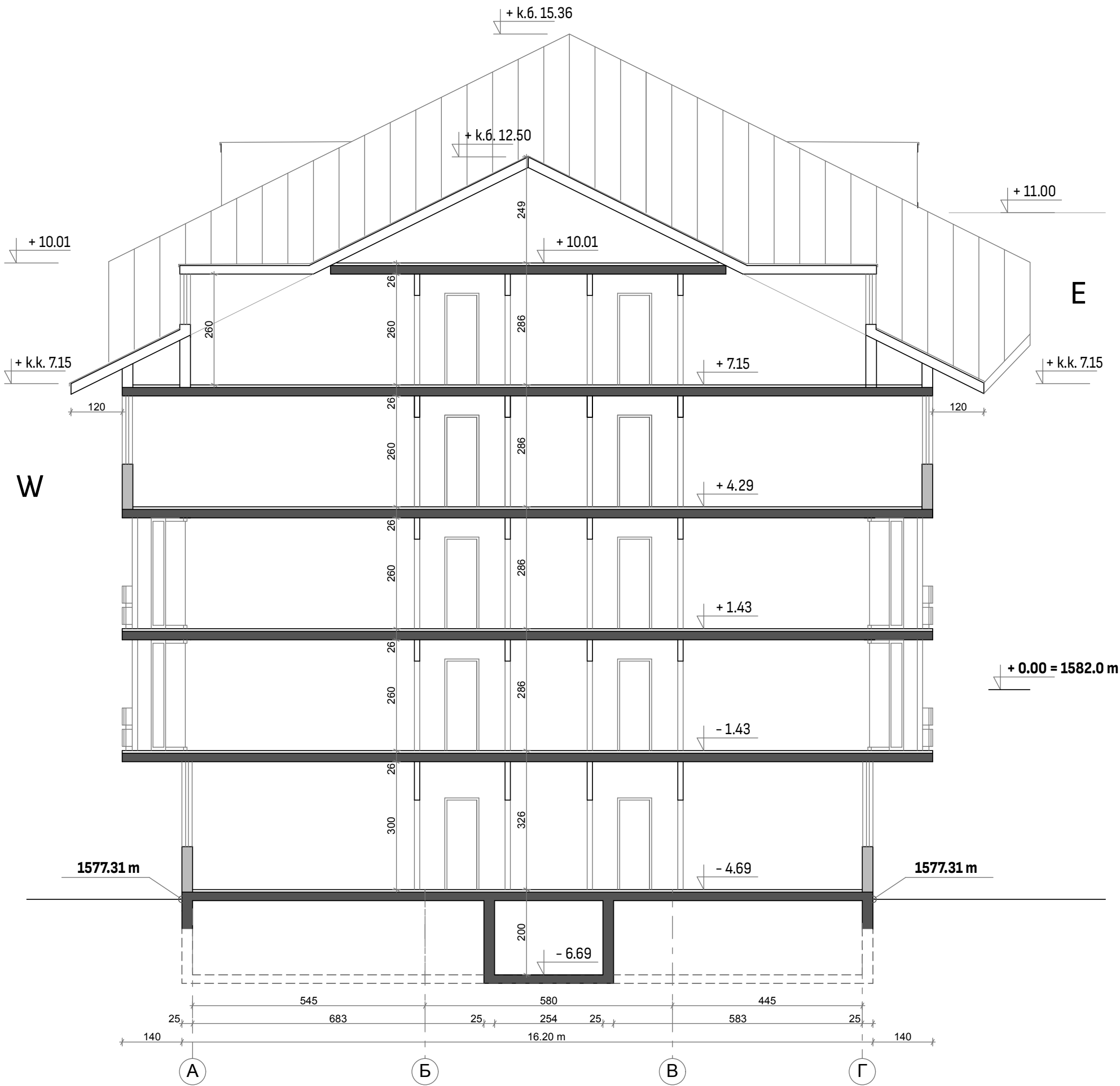
БЛОК А Разрез А - А М1:100
