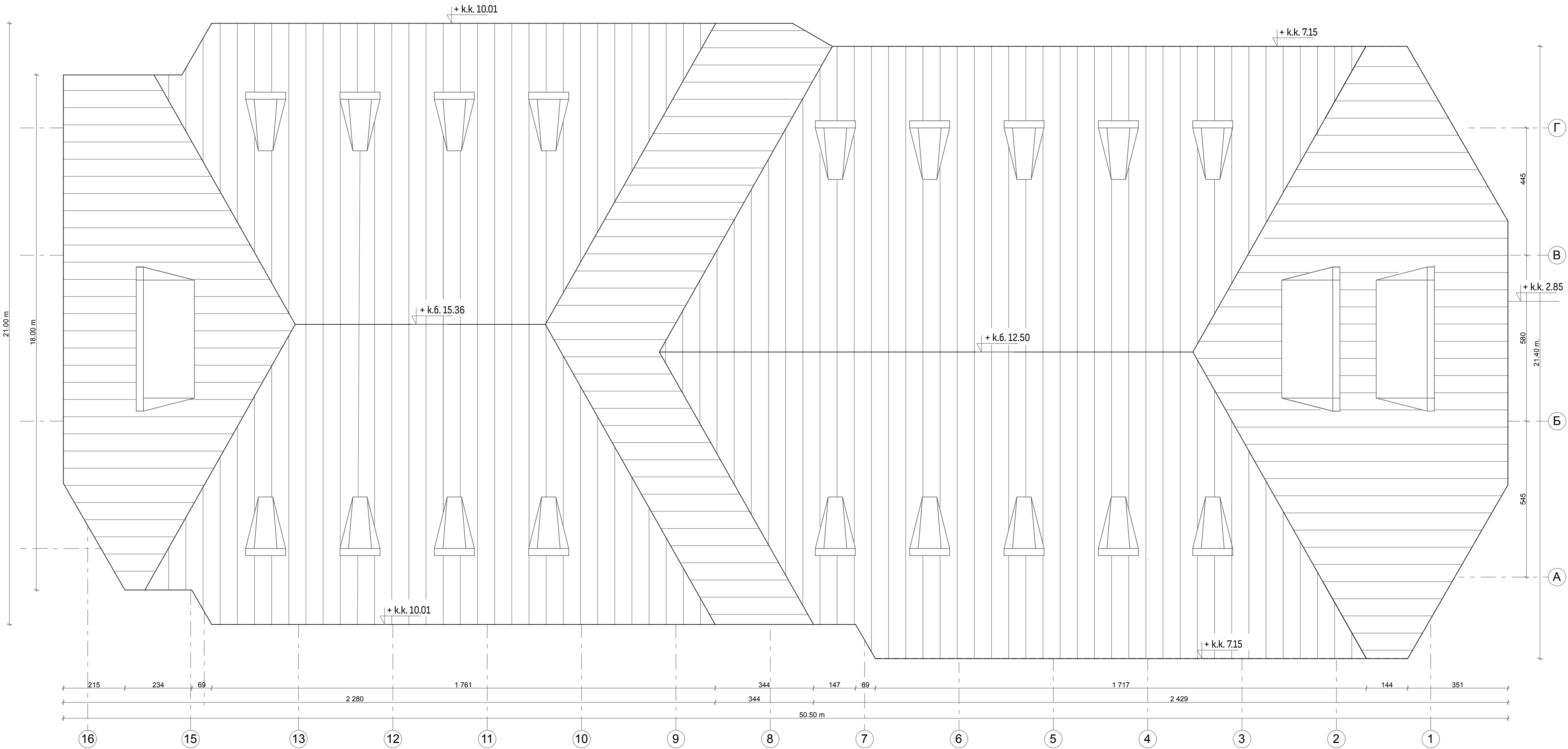
БЛОК А План на покрива М1:100
