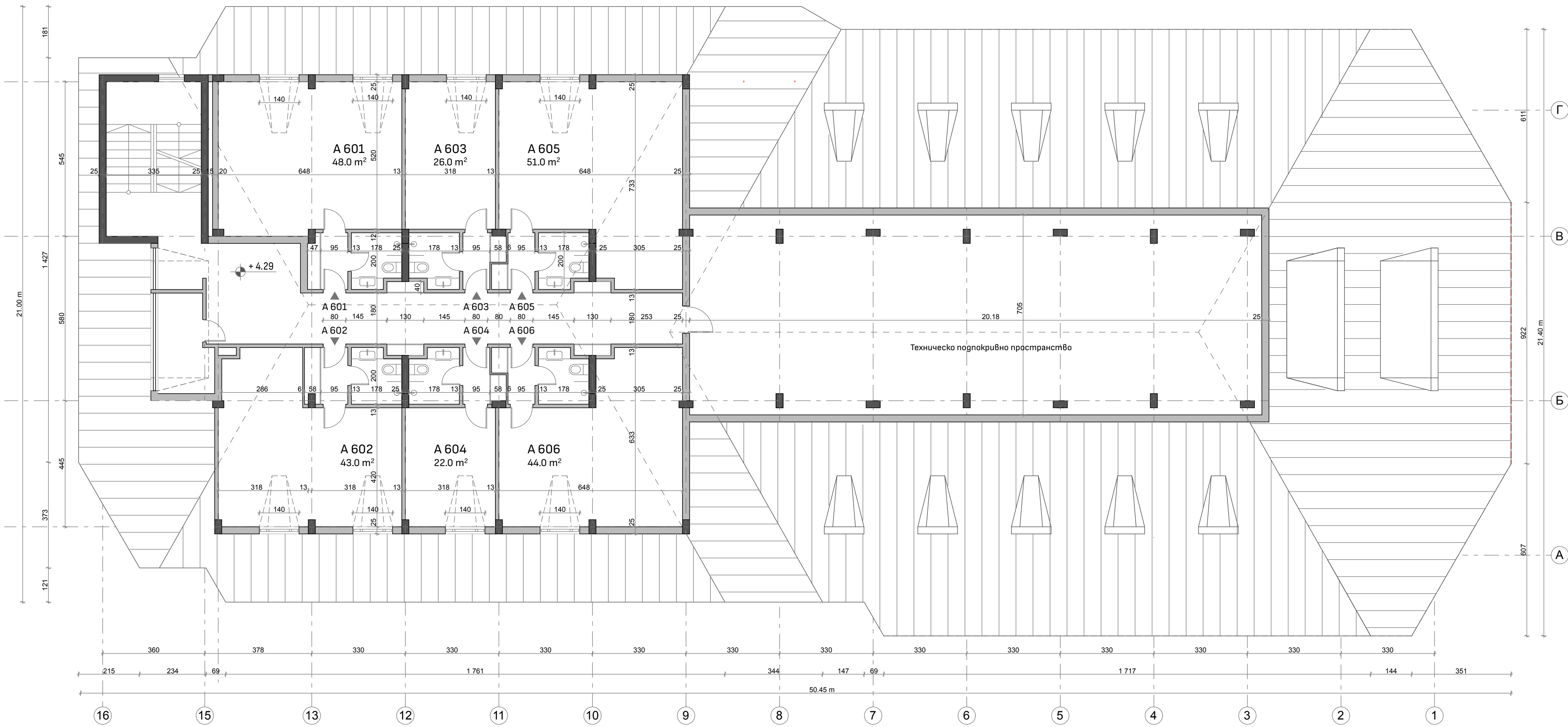
БЛОК А Разпределение на пети подпокривен етаж М 1 : 100 + 10.01
