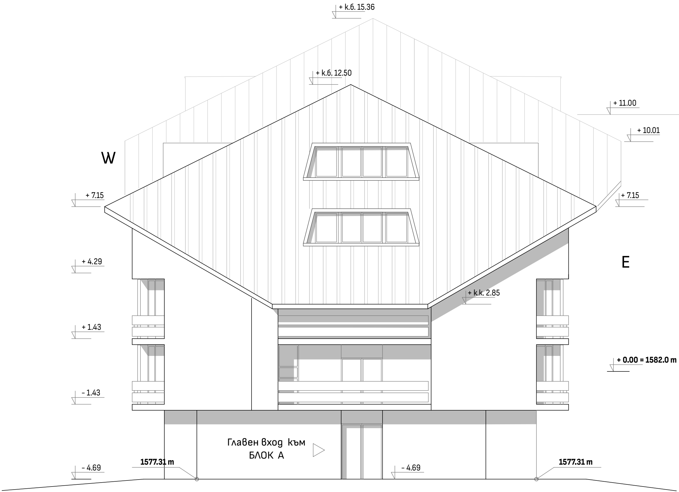
Югозападна фасада М1:100
